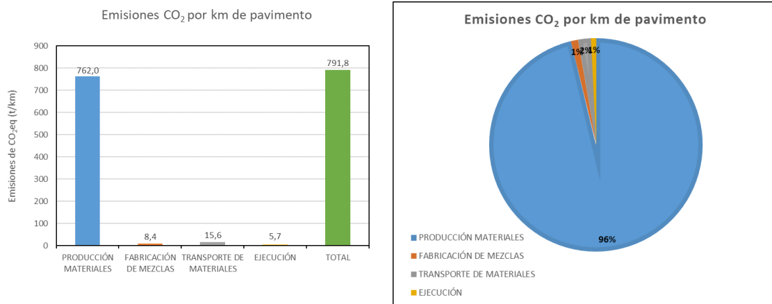
Figura 12: Emisiones de CO 2eq según Etapas del Ciclo de Vida Tramo 2 Proyecto Tegucigalpa- La Venta (Aldea Santa Rosa – Cerro de Hula)
