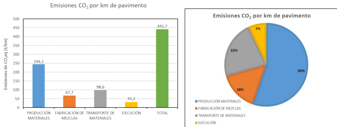
Figura 2: Emisiones de CO 2 eq según etapas del ciclo de vida para el tramo 1 Proyecto Arica– Tambo Quemado Fuente: Elaboración propia
