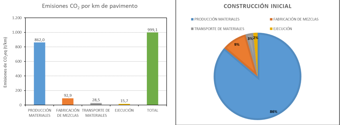
Figura 18: Emisiones de CO 2eq según etapas del ciclo de vida Tramo 3 – Subtramo 2 Proyecto Tegucigalpa- La Venta Fuente: Elaboración propia
