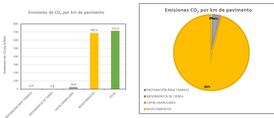
Figura 11: Emisiones de CO 2 eq según procedimientos de construcción Tramo 1 Proyecto Tegucigalpa- La Venta (Tegucigalpa - Desvío Aldea Santa Rosa) Fuente: Elaboración propia
