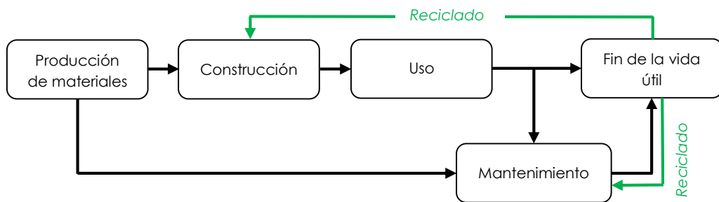
Figura 1: Ciclo de vida de un Camino pavimentado Fuente: Elaboración propia
