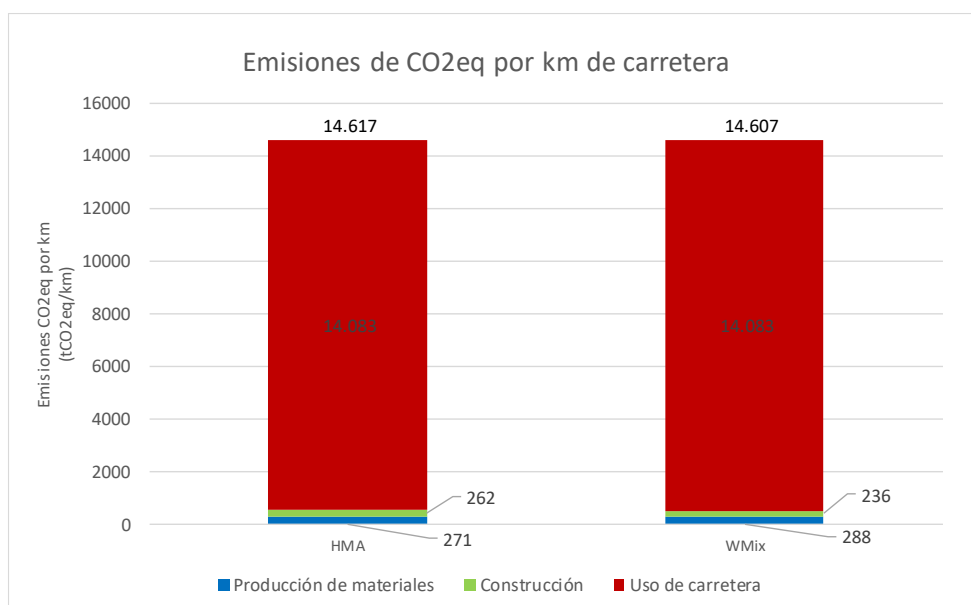
Figura RE 3: Emisiones de CO 2 eq por km para HMA y WMix, según fase Proyecto Lo Orozco-Quilpué
