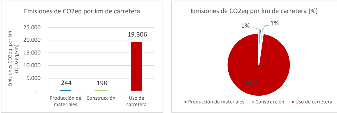
Figura 6: Emisiones de CO 2eq por km para Proyecto Arica- Tambo quemado según fases Fuente: Elaboración propia
