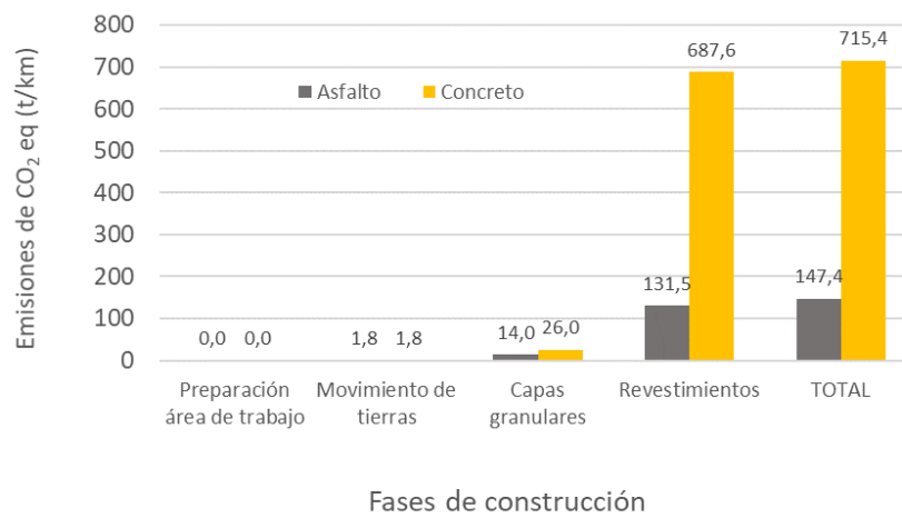
Figura 28: Emisiones de CO 2eq por km según las fases de construcción para el tramo 1
