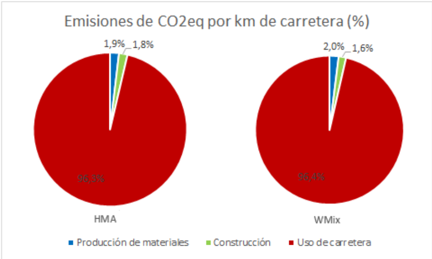
Figura 26: Emisiones de CO 2 eq por km porcentuales para HMA y WMix, según fase Proyecto Lo Orozco- Quilpué Fuente: Elaboración propia
