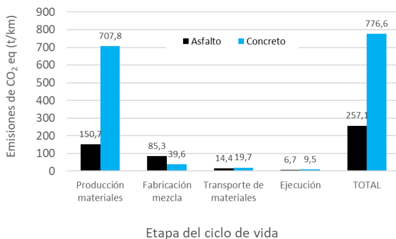
Figura 31: Emisiones de CO 2eq por km según etapa del ciclo de vida para el tramo 3
