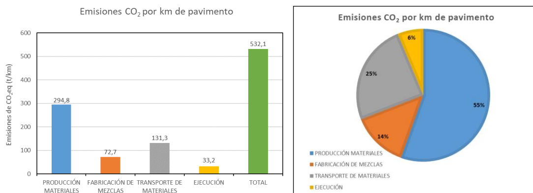
Figura 7: Emisiones totales de CO 2eq según etapas del ciclo de vida Proyecto Alto Chiza - Cuya Fuente: Elaboración propia
