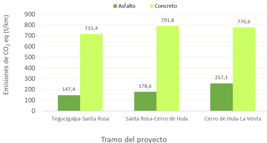
Figura 33: Emisiones de CO 2eq por km para los tres tramos y cada tipo de pavimento
