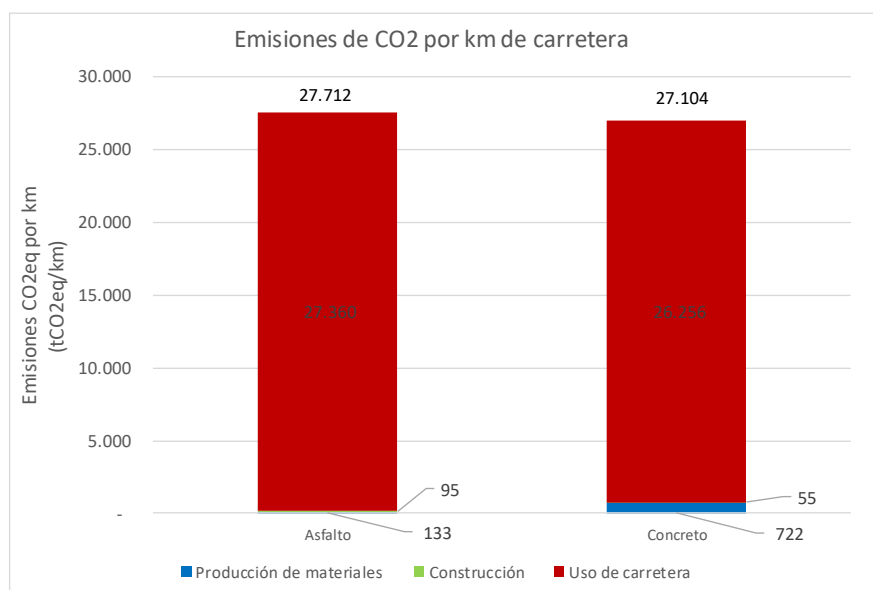
Figura RE 4: Emisiones de CO 2 para asfalto y concreto según fase Proyecto Tegucigalpa- La Venta, Asfalto Fuente: Elaboración propia
