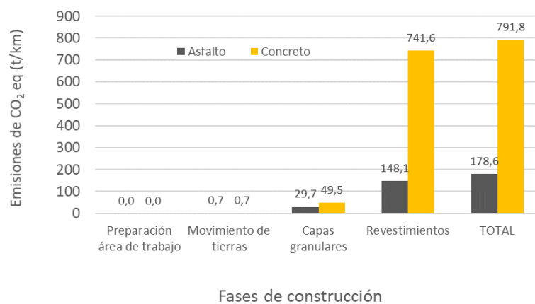
Figura 30: Emisiones de CO 2 eq por km según las fases de construcción para el tramo 2
