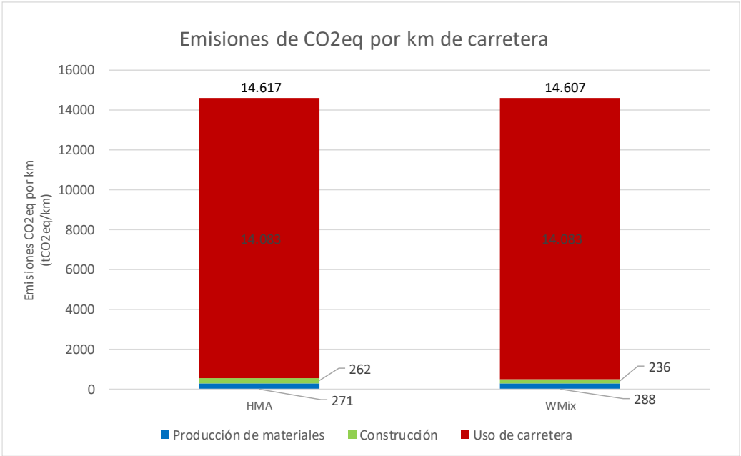
Figura 25: Emisiones de CO 2 eq por km para HMA y WMix, según fase Proyecto Lo Orozco- Quilpué Fuente: Elaboración propia
