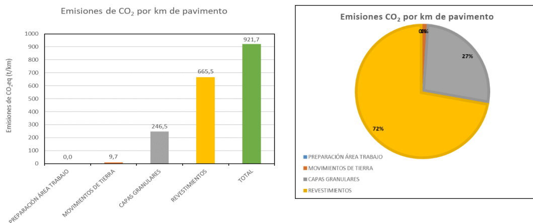
Figura 16: Emissiones de CO 2 eq según procedimientos de construcción Tramo 3 – Subtramo 1 Proyecto Tegucigalpa- La Venta Fuente: Elaboración propia
