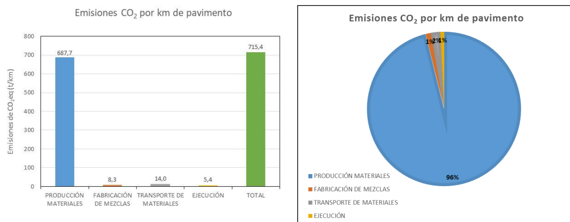
Figura 10: Emisiones de CO 2 eq según etapas del ciclo de vida Tramo 1 Proyecto Tegucigalpa- La Venta (Tegucigalpa - Desvío Aldea Santa Rosa) Fuente: Elaboración propia
