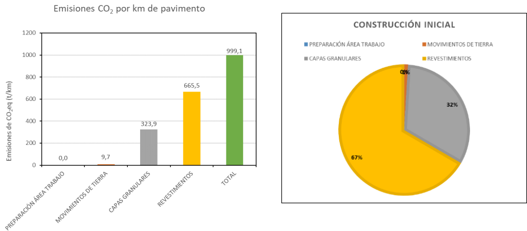
Figura 19: Emisiones de CO 2eq según procedimientos de construcción Tramo 3 – Subtramo 2 Proyecto Tegucigalpa- La Venta Fuente: Elaboración propia
