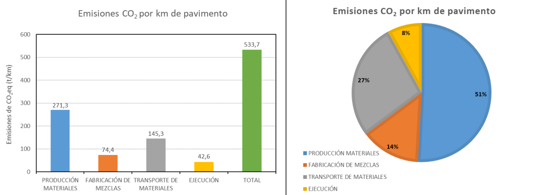
Figura 21: Emisiones totales de CO 2 eq según ciclo de vida para estructura con mezcla asfáltica en caliente (HMA) proyecto Lo Orozco - Quilpué
