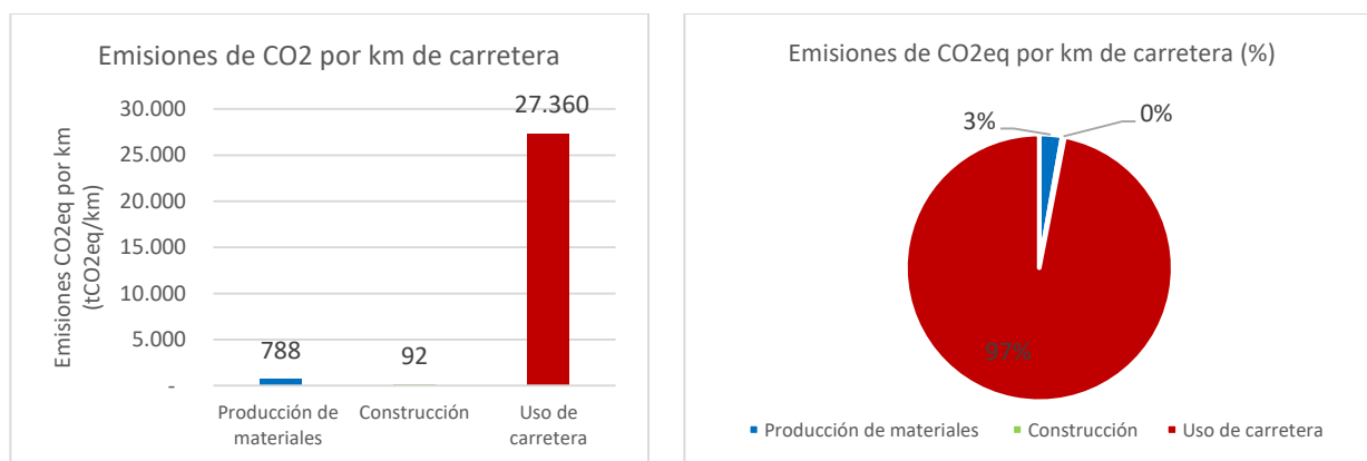
Figura 20: Emisiones de CO 2eq por km según fase Proyecto Tegucigalpa- La Venta
