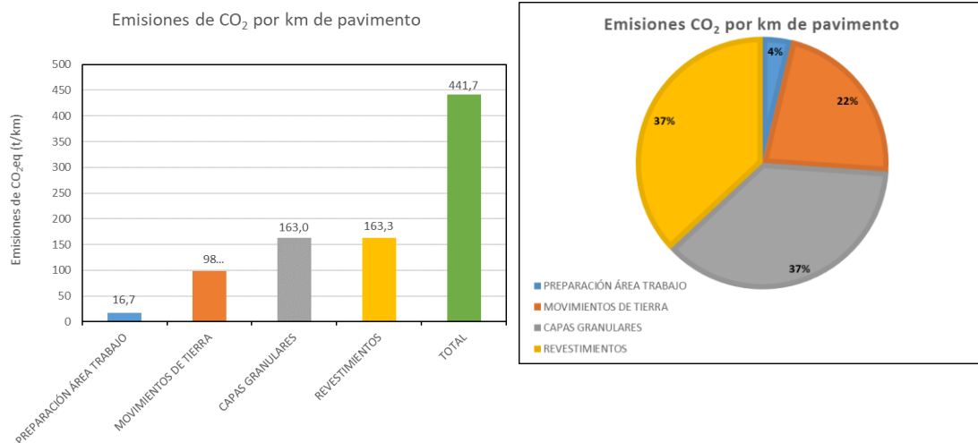
Figura 3: Emisiones de CO 2 eq según procedimientos de construcción para el tramo 1 Proyecto Arica– Tambo Quemado Fuente: Elaboración propia
