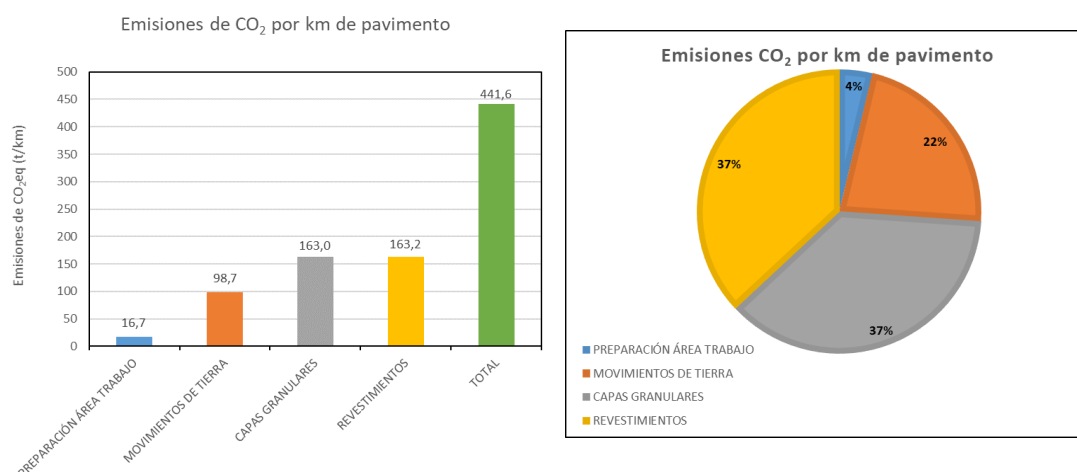
Figura 5: Emisiones de CO 2 eq según procedimientos de construcción para el tramo 2 Proyecto Arica– Tambo Quemado Fuente: Elaboración propia
