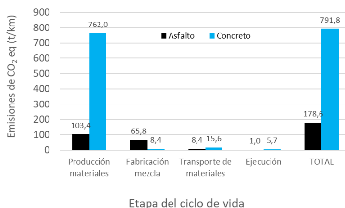
Figura 29: Emisiones de CO 2eq por km según etapa del ciclo de vida para el tramo 2
