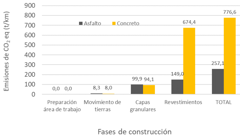
Figura 32: Emisiones de CO 2eq por km según las fases de construcción para el tramo 3
