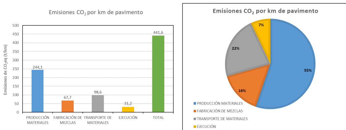
Figura 4: Emisiones totales de CO 2 eq según etapas del ciclo de vida para el tramo 2 Proyecto Arica– Tambo Quemado Fuente: Elaboración propia
