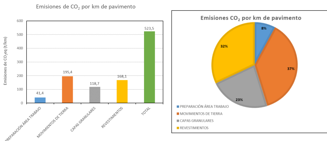
Figura 24: Emisiones totales de CO 2 eq según procedimientos de construcción para estructura con mezcla asfáltica tibia (WMix) Fuente: Elaboración propia
