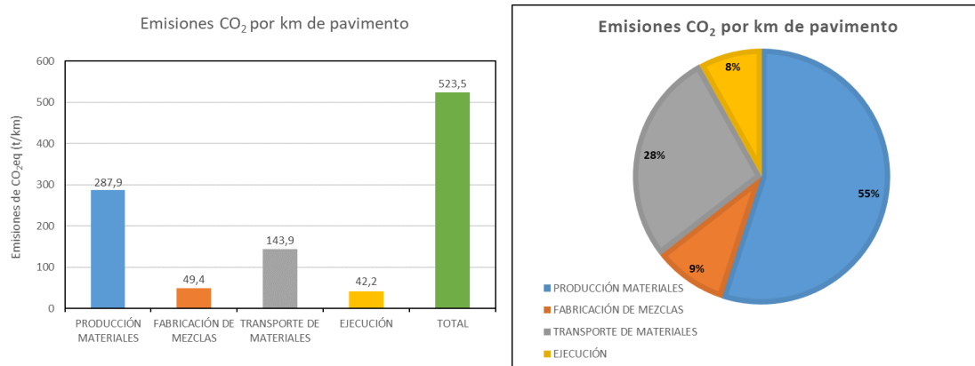
Figura 23: Emisiones totales de CO 2 eq según las etapas del ciclo de vida para estructura con mezcla asfáltica tibia (WMix) Fuente: Elaboración propia
