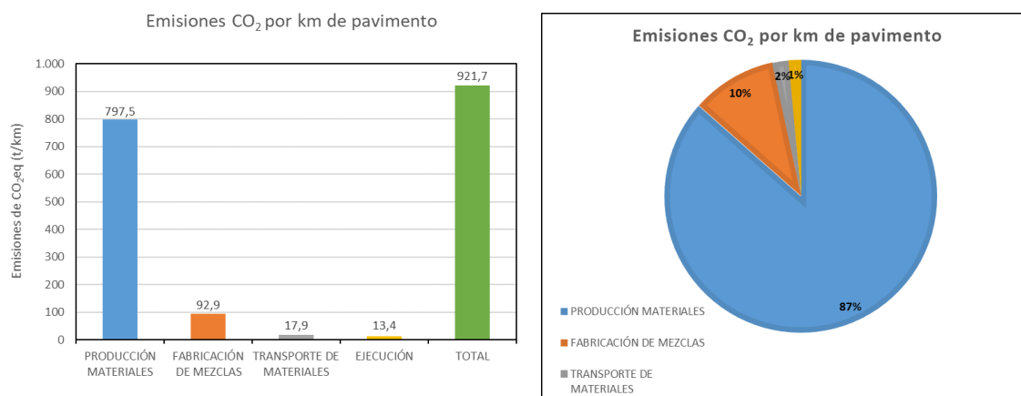
Figura 15: Emisiones de CO 2eq según etapas del ciclo de vida Tramo 3 – Subtramo 1 Proyecto Tegucigalpa- La Venta Fuente: Elaboración propia
