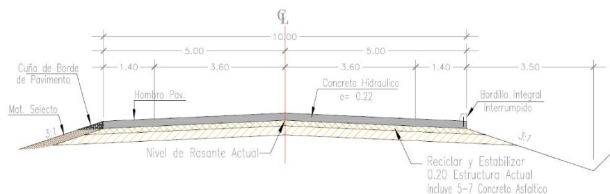
Figura 14: Sección transversal tipo para el tramo Dm 17.500 – Dm 43.900
