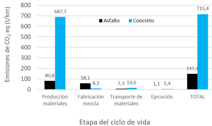
Figura 27: Emisiones de CO 2eq por km según etapa del ciclo de vida para el tramo 1
