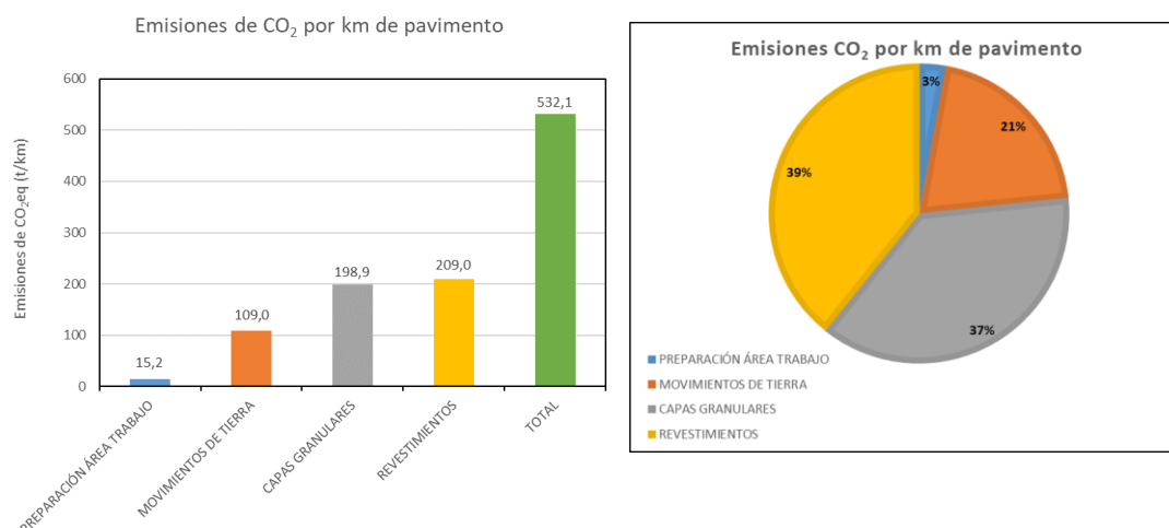
Figura 8: Emisiones totales de CO 2 eq según procedimientos de construcción Proyecto Alto Chiza - Cuya
