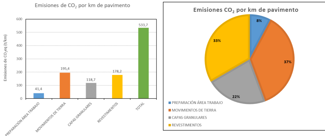
Figura 22: Emisiones totales de CO 2 eq según procedimientos de construcción para estructura con mezcla asfáltica en caliente (HMA) proyecto Lo Orozco - Quilpué Fuente: Elaboración propia
