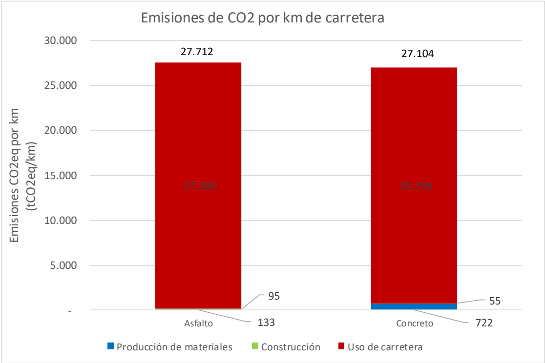
Figura 34: Emisiones de CO 2 para asfalto y concreto según fase Proyecto Tegucigalpa- La Venta, Asfalto
