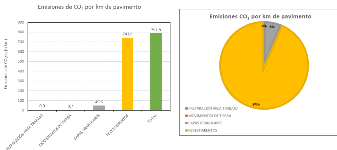
Figura 13: Emissiones de CO 2 eq según procedimientos de construcción Tramo 2 Proyecto Tegucigalpa- La Venta (Aldea Santa Rosa – Cerro de Hula) Fuente: Elaboración propia
