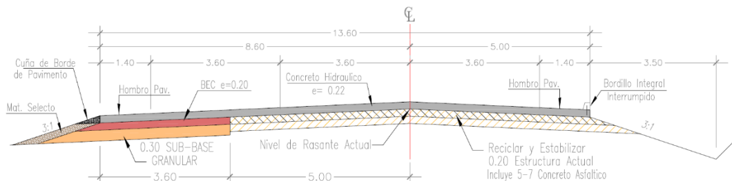
Figura 17: Sección transversal tipo para el tramo Dm 17.500 – Dm 43.900
