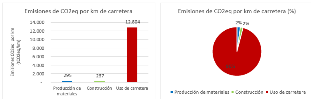
Figura 9: Emisiones de CO 2 eq por km para Proyecto Alto Chiza- Cuya según fases Fuente: Elaboración propia
