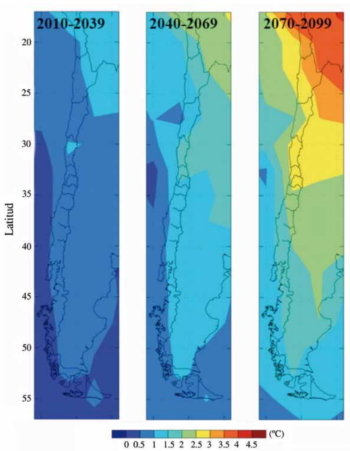
FIGURA 1.2 CHILE: PROYECCIONES DE TEMPERATURA PARA EL ESCENARIO B2 (Cambios en grados centígrados sobre base histórica)
