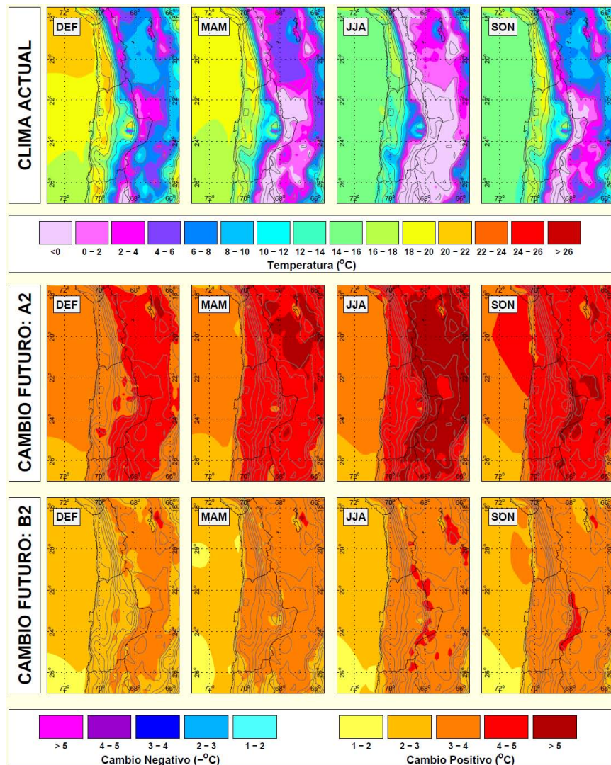
Figura 2. Proyección de cambio de temperaturas en el Norte de Chile en base al modelo PRECIS-HadCM3. En la parte superior: Temperatura media en DEF, MAM, JJA Y SON, para el periodo 1961-1990. En la parte media e inferior: Cambio en temperatura entre los periodos 1961-1990 y 2071-2100 para los escenarios A2 y B2, respectivamente. (Fuente: DGF-CONAMA, 2008)
