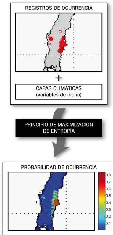
Figura 4. Esquema representativo del método de máxima entropía.
