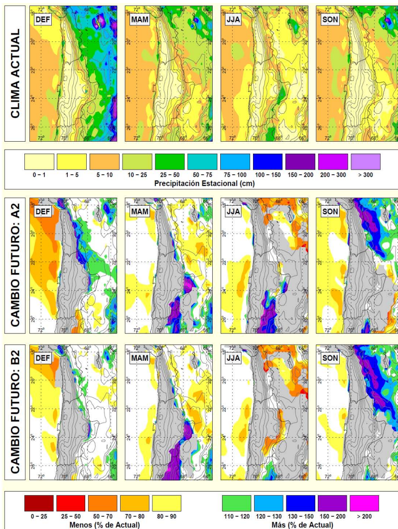
Figura 3. Proyección de cambio de precipitación en el norte de Chile en base al modelo PRECIS-HadCM3. En la parte superior: Precipitación total en DEF, MAM, JJA Y SON, para el periodo 1961-1990. En la parte media e inferior: Cambio en precipitaciones entre los periodos 1961-1990 y 2071-2100 para los escenarios A2 y B2, respectivamente. (Fuente: DGF-CONAMA, 2008)
