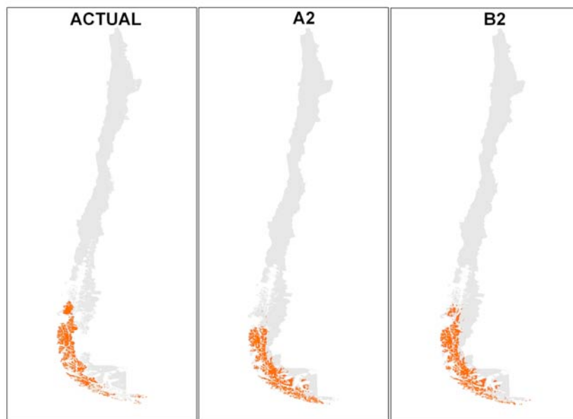
Figura 37. Turberas: No presenta variaciones relevantes en su rango de distribución actual, solamente en el escenario A2 se observa una leve disminución en su límite de distribución norte.
