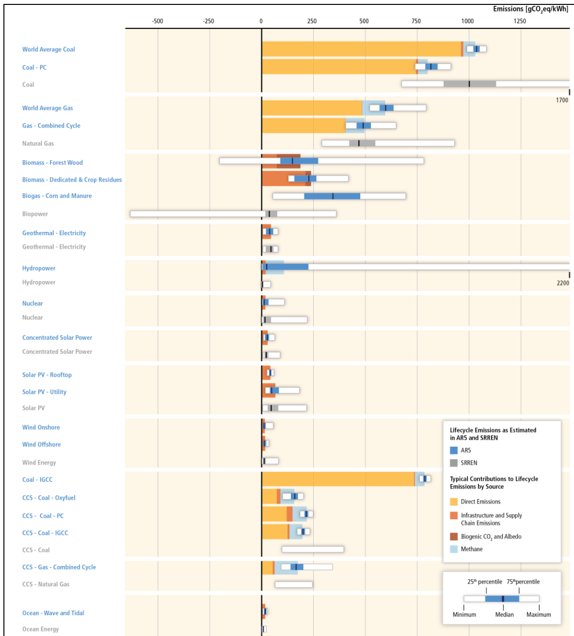
Figura 3. Factores de emisión de Tecnologías de generación de electricidad (Bruckner et al., 2014 / IPCC AR5)
