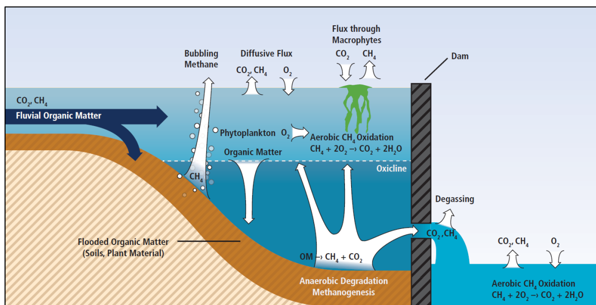
Figura 4. Emisiones brutas de GEI desde embalses (Kumar et al., 2011)
