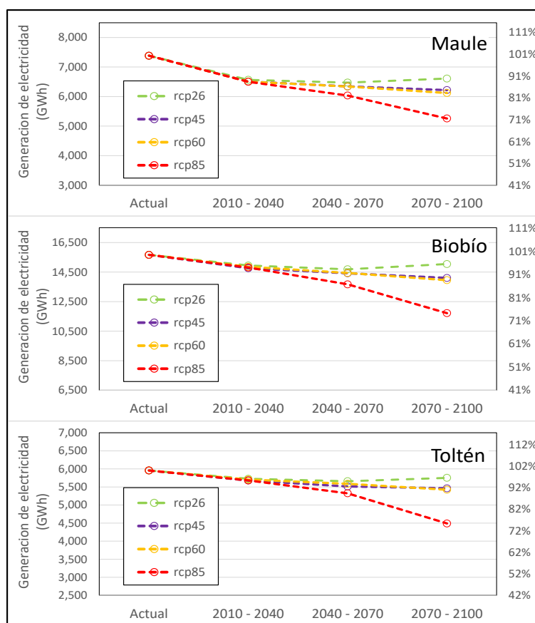
Figura 1. Potencial de generación hidroeléctrica futura en cuencas Maule, Biobío y Toltén (Proyecto Cuencas. Ministerio de Energía, 2016)
