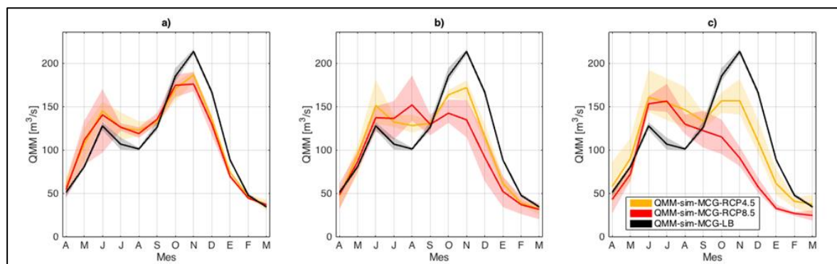
Figura 2. Caudales medios mensuales en subcuenca del Rio Melado para un escenarios histórico y distintos escenarios de emisión de GEI para los periodos a) 2009-2039; b) 2039-2069 y c) 2069-2099 (Ministerio de Energía 2016b).
